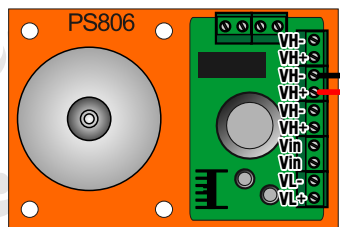
Линейный источник питания Leadshine PS806-12
