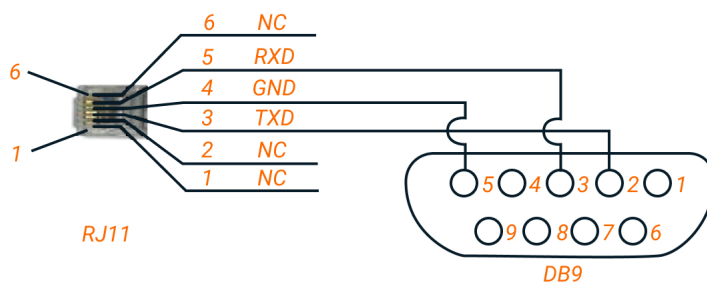
Конфигурация интерфейса RS232 драйвера EM882S
