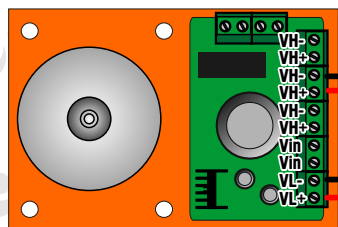
Линейный источник питания Leadshine PS408-12
