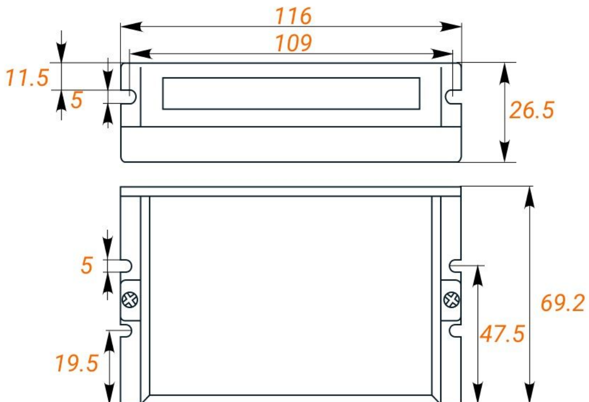
Рис. 1. Габаритные размеры серводрайвера CS-D508
