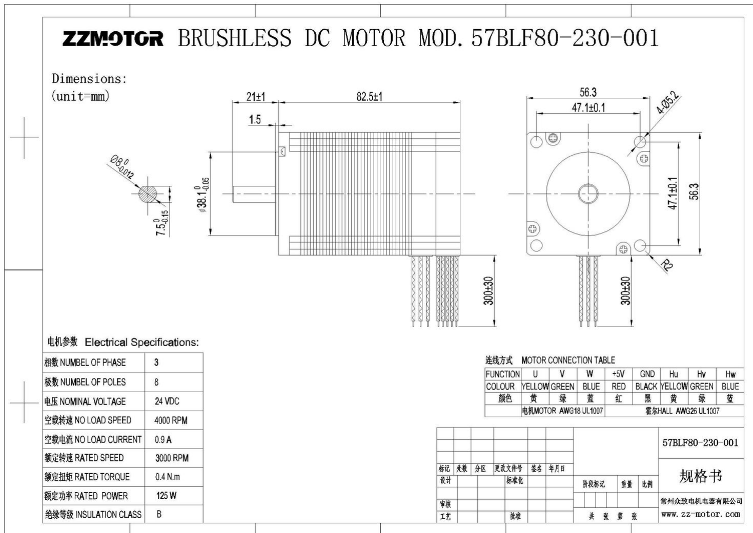
Рис. 1. Габаритные размеры 57BLF80-230
