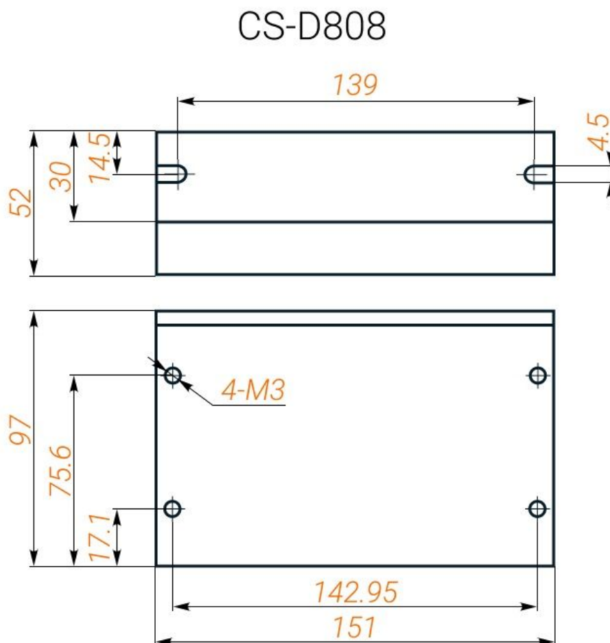
Рис. 1. Габаритные размеры серводрайвера CS-D808
