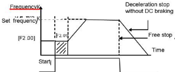
Рисунок 6-12 Выходная кривая стартовой частоты и частоты останова
