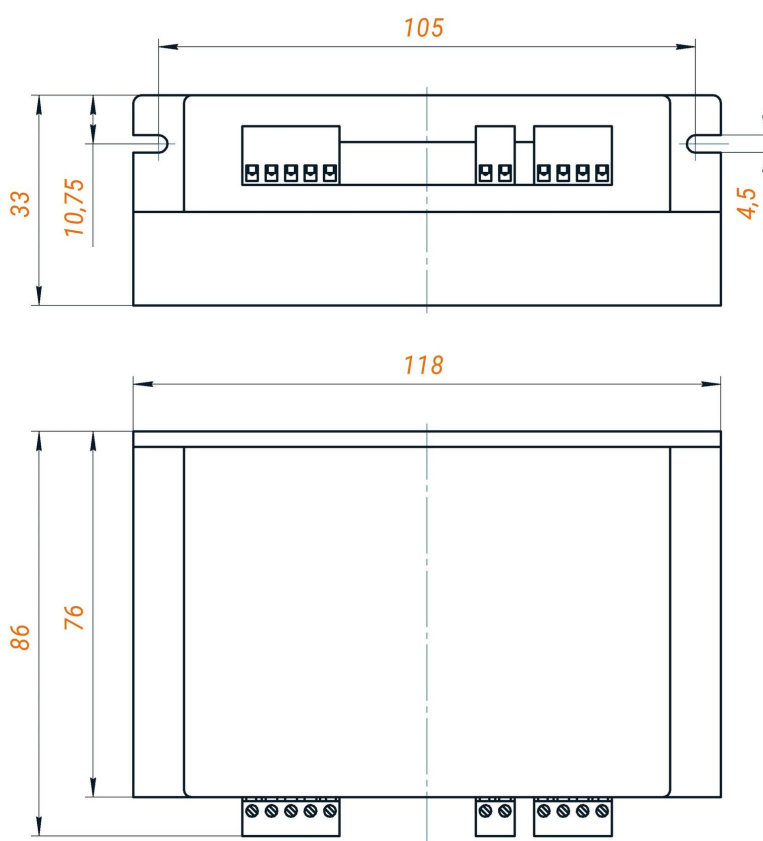
Рис. 1. Габаритные размеры драйвера YKD2405M-DS
