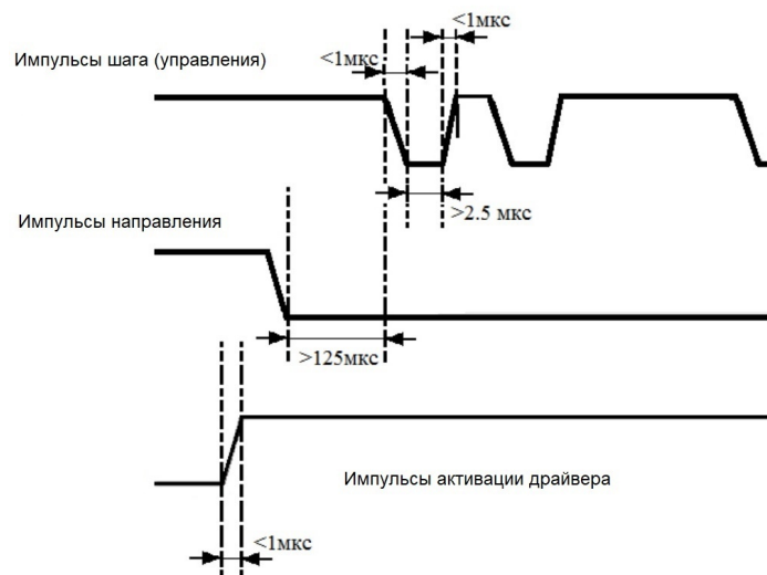
Рис. 3. Временные диаграммы входных сигналов
