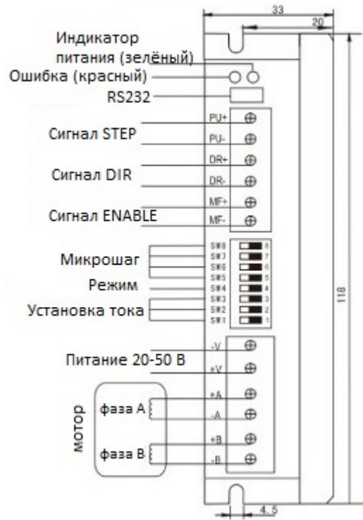
Рис. 2. Схема подключения драйвера YKD2608MN
