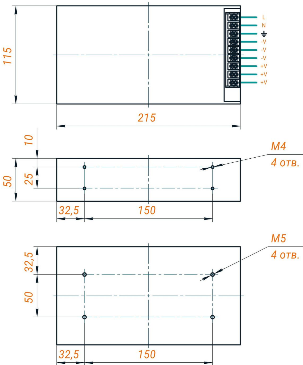
Рис. 1. Габариты и распиновка источника питания S-350
