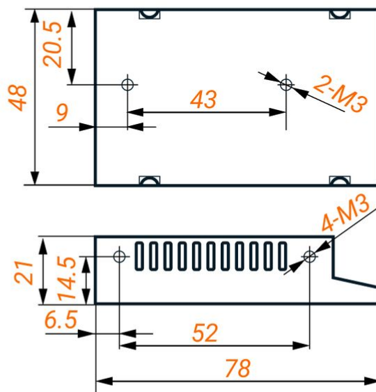
Рис. 1. Габариты и распиновка источников питания MSF-10
