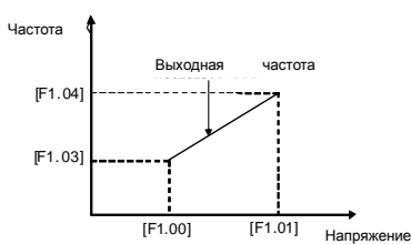
Рисунок 6-6. Иллюстрация соотношения между входной аналоговой величиной и заданной частотой
