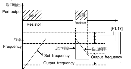
Рисунок 6-9 Сигнал приближения к частоте
