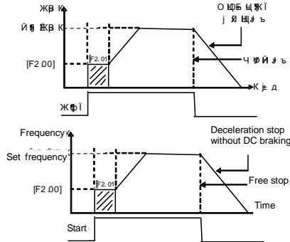
Рисунок 6-12 Выходная кривая стартовой частоты и частоты остановки
