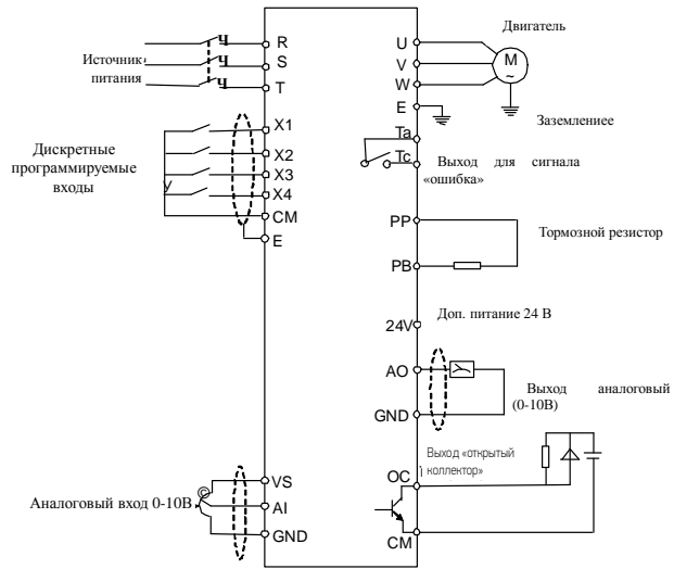
Рисунок 3-3. Стандартная схема подключения преобразователя
