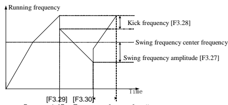
Рисунок 6-17 Процесс работы рабочей частоты
