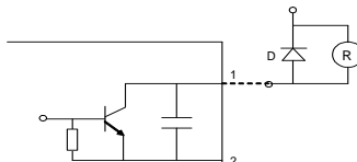
Рисунок 6-8. Внутренняя цепь выходного терминала ОК
