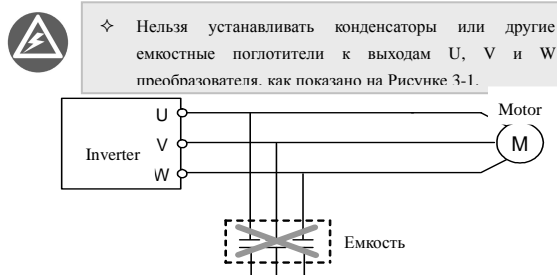
Рисунок 3-1. Запрет на подключение фильтрующего конденсатора
