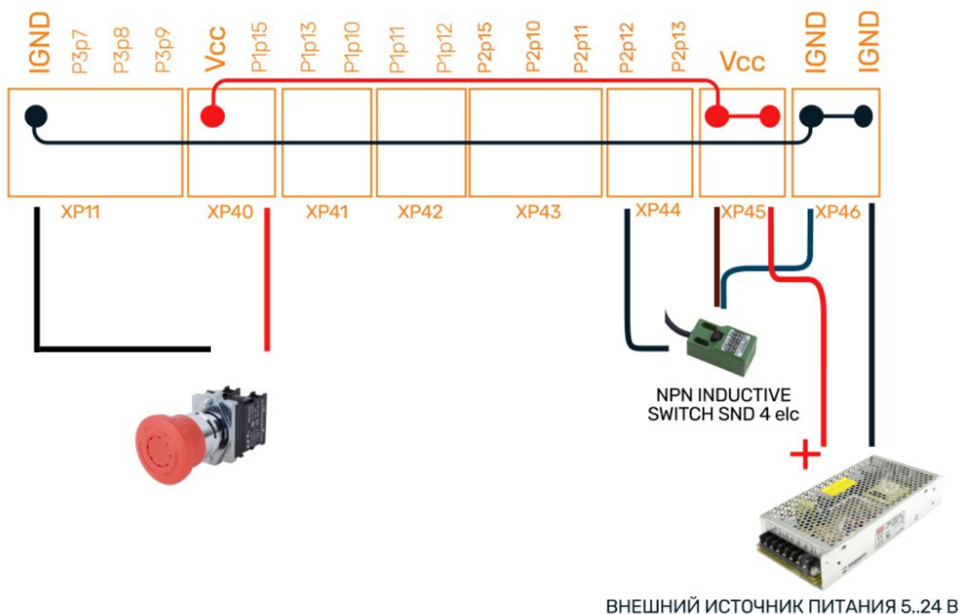
Рис. 5. Пример подключения датчиков к DX106
