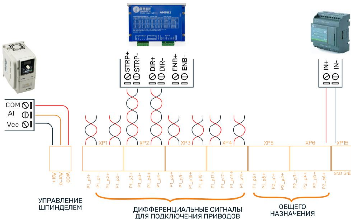
Рис. 1. Подключение устройств к выходам DX106
