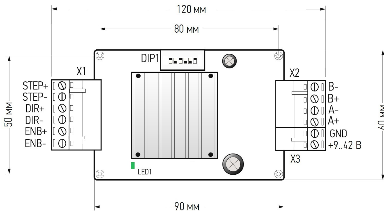
Рис. 1. Габаритные размеры и распиновка драйвера STB42-1
