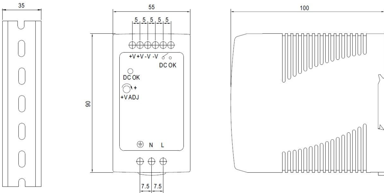
Рис. 1. Габариты и распиновка источников питания MDR-100
