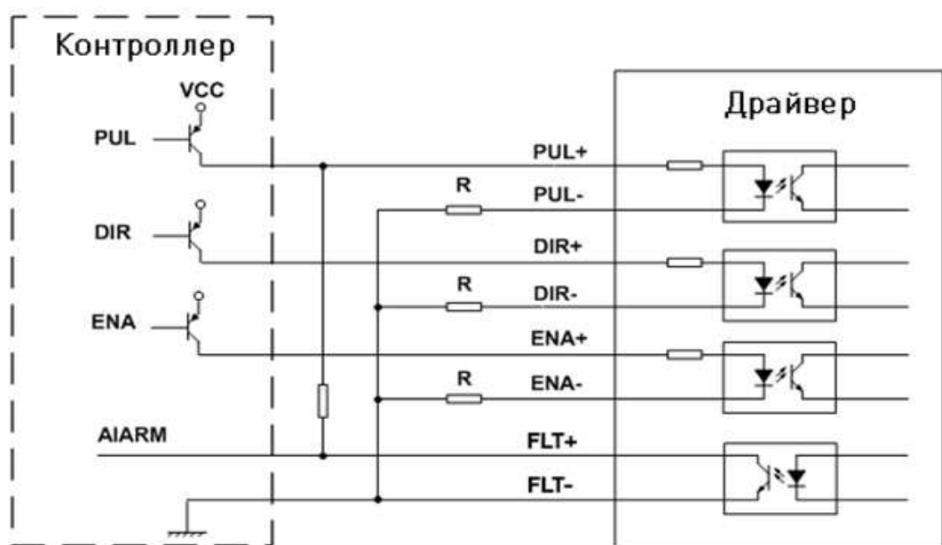
Рис 2. Подключение с общим катодом
